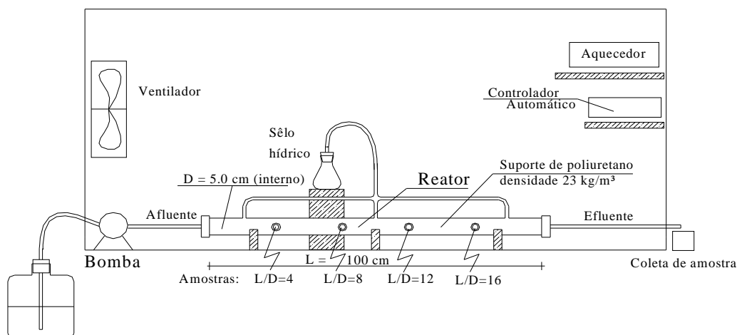
Figura 1 – Reator Anaeróbio Horizontal de Leito Fixo utilizado para o tratamento de formol
